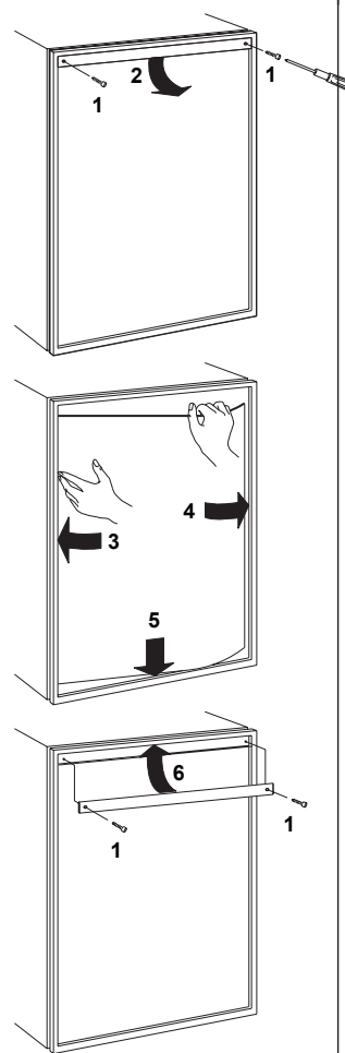
FIG 28 - DOOR PANEL
